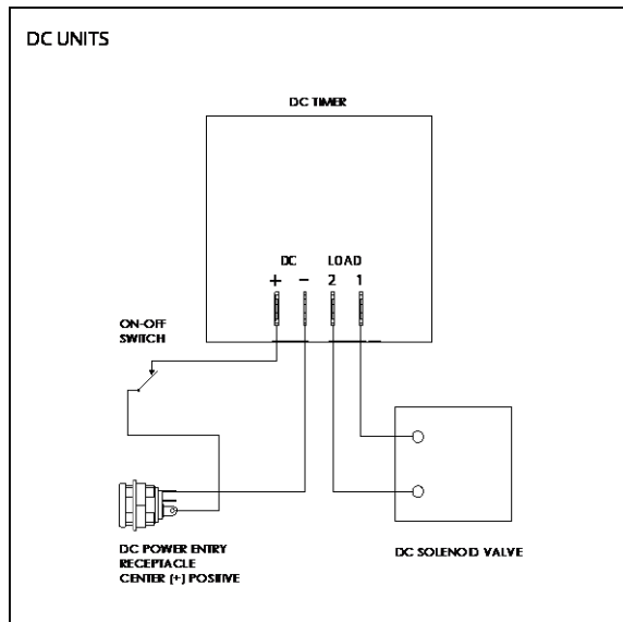
CO2-PG14 WIRING DIAGRAM
